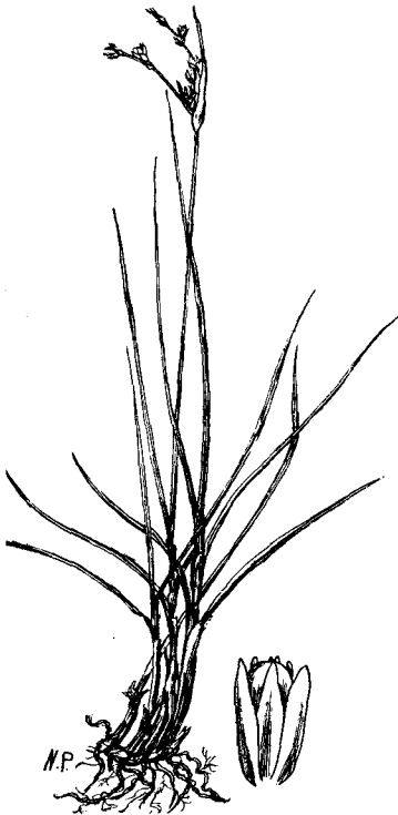
FIG. 707. — Juncus compressus .
