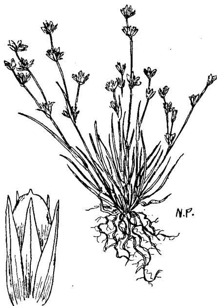
FIG. 719. — Juncus bulbosus .
